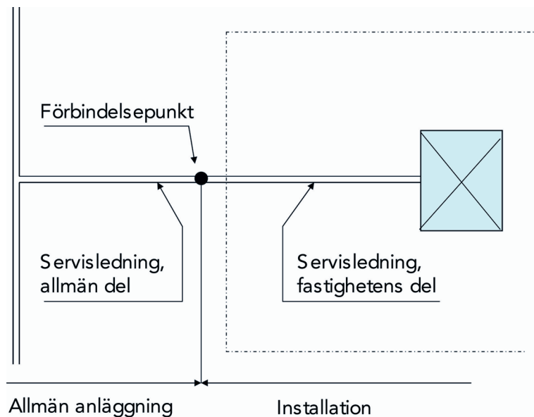
Figur 1. Uppdelning i allmän Va-anläggning och fastighetsägarens VA-installation
